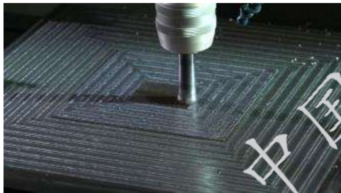
CNC数控加工
